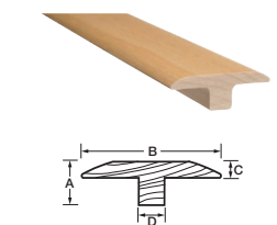
Moulure en T
