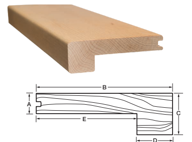
Nez de marche carré
