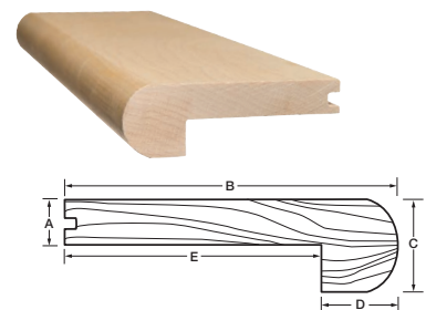
Nez de marche rond
