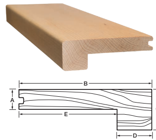
Nez de marche carré
