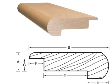
Nez de marche rond (Installation non fixée)
